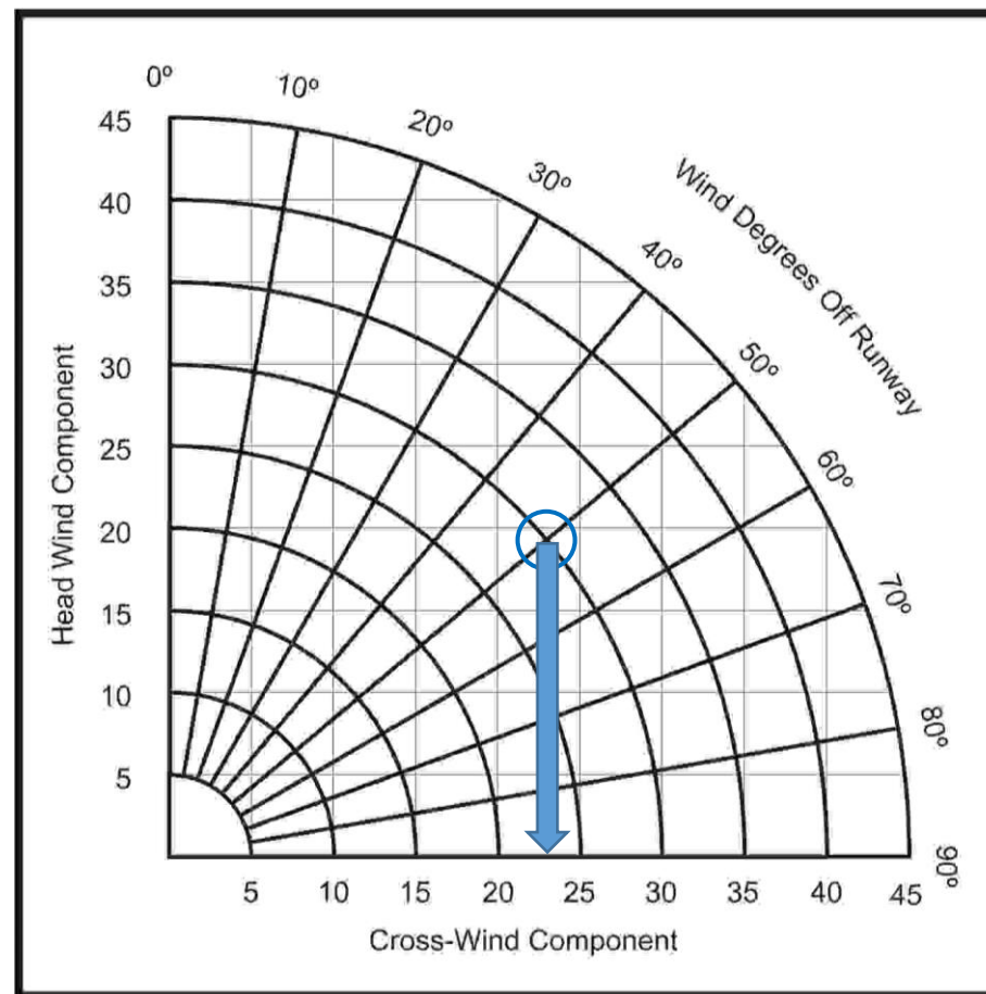
Exemple: RWY 36 - Wind 050/30kts Composante de vent de travers 23kts
